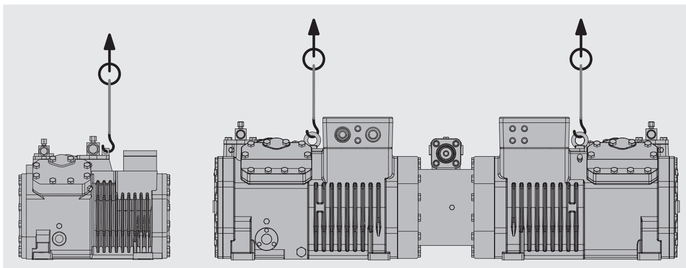
Abb. 1 Verdichter anheben
