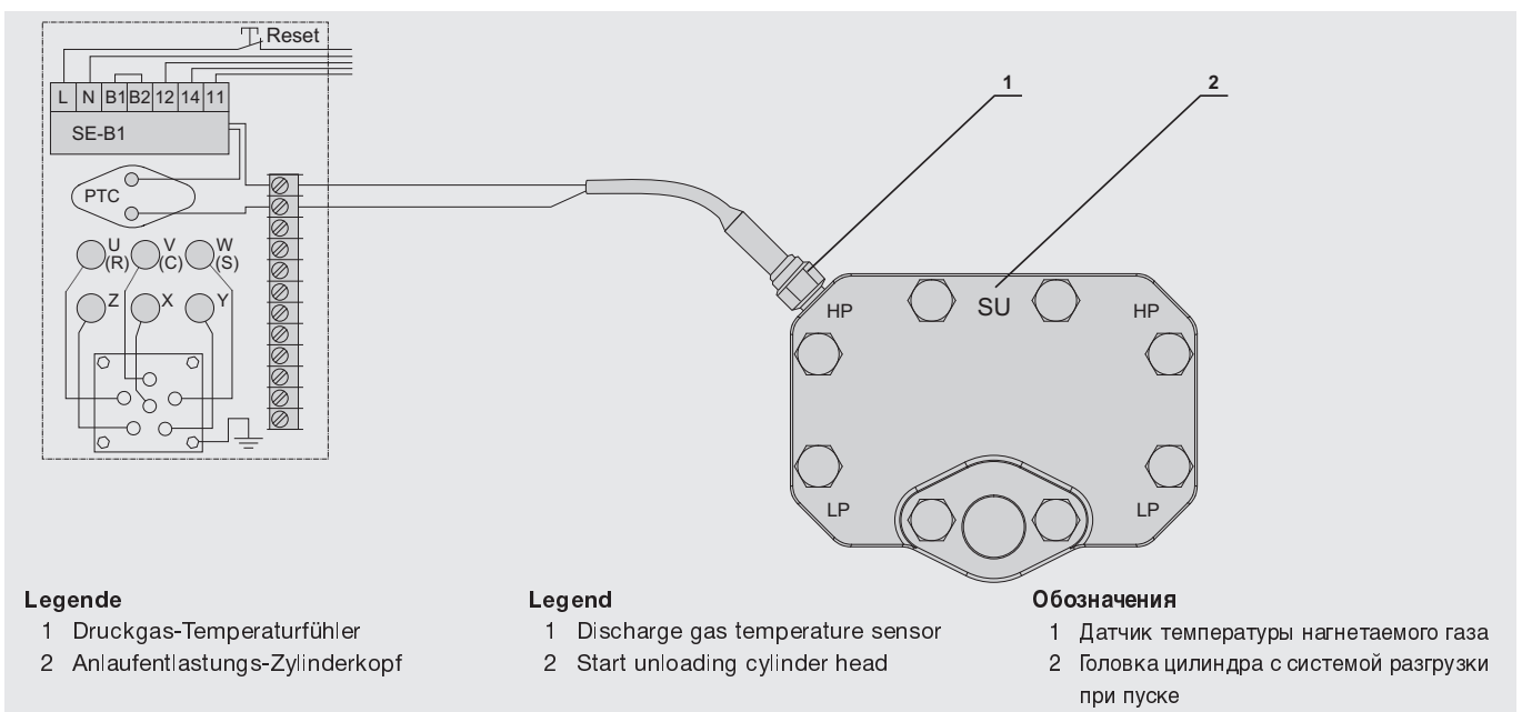
Abb. 6 Druckgas-Temperaturfühler anschließen
