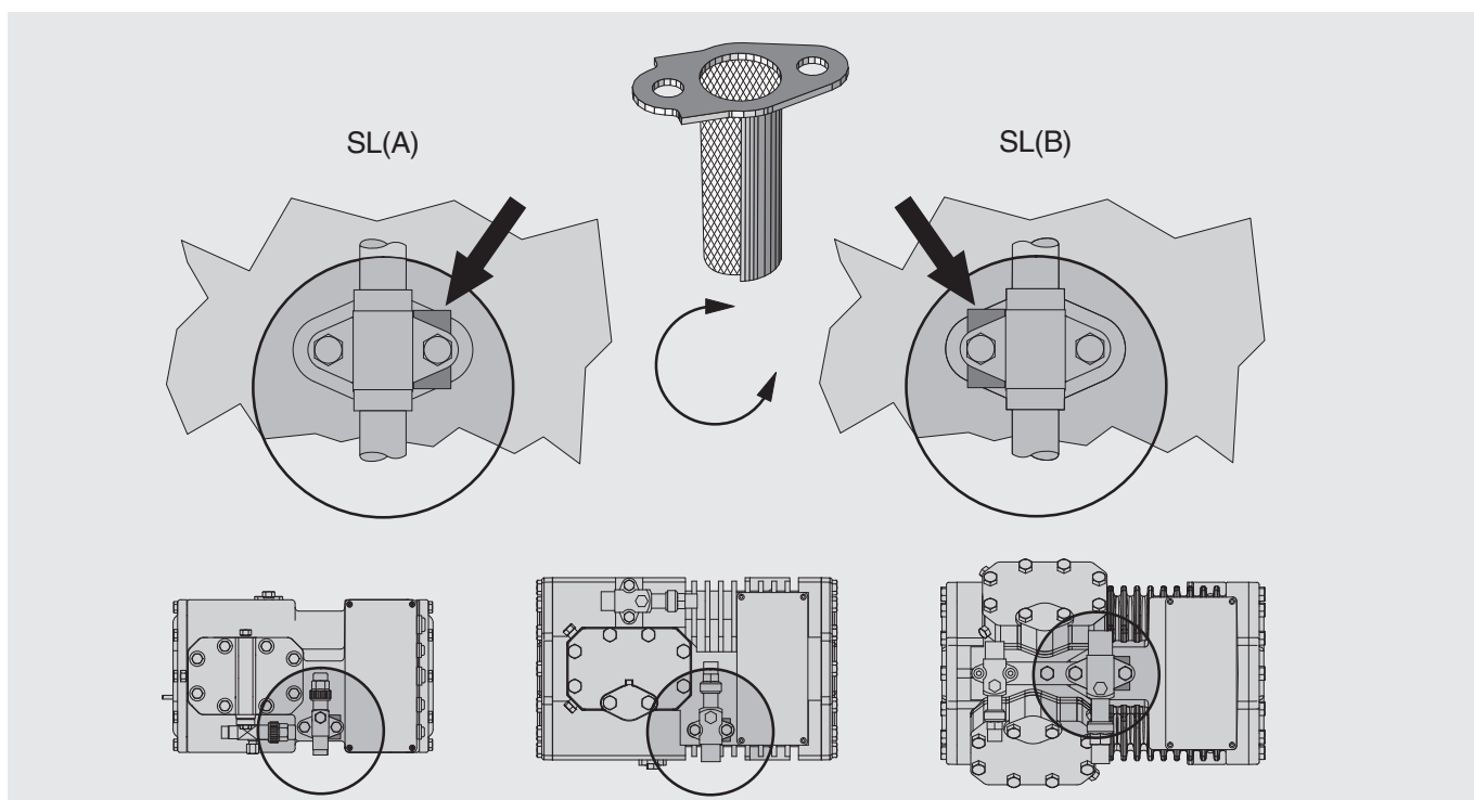
Abb. 5 VARICOOL-System
