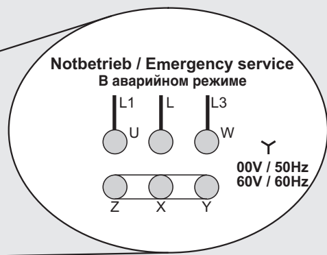
Рис.12 LHV5E/2DES-3.F1Y: Наклейка в крышке клеммной коробки компрессора (тип компрессора CE2)
