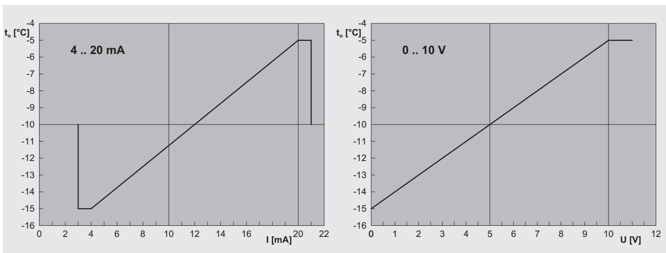
Abb. 6 Stufenlose Saugdruckanhebung über Sollwertjustierung Beispiel: -10^{\circ}\text{C} (Sollwert) und 5,0\text{ K} (Abweichung) eingestellt.
