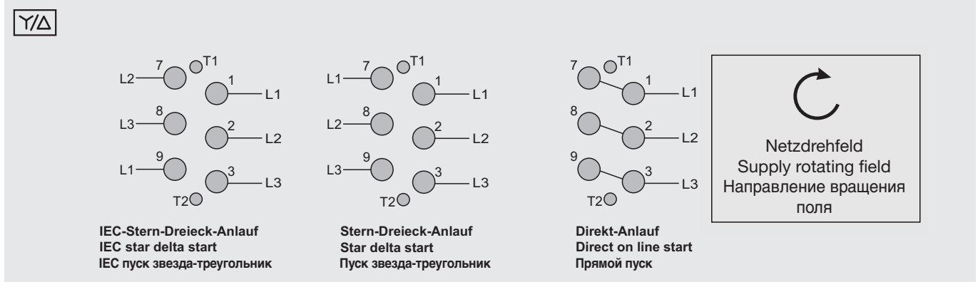
Abb. 22 Motoranschluss (Y/Δ)
