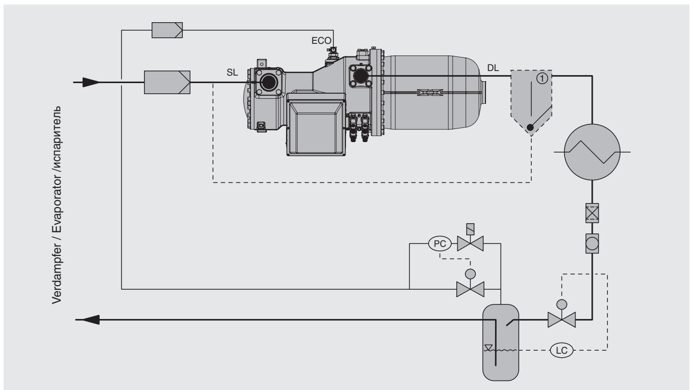
Abb. 16 ECO-System mit Mitteldrucksammler ① Sekundär-Ölabscheider bei Systemen mit überflutetem Verdampfer
